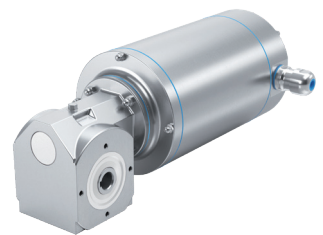
Schneckengetriebe SMN mit Edelstahlmotor SBH mit IP69K
